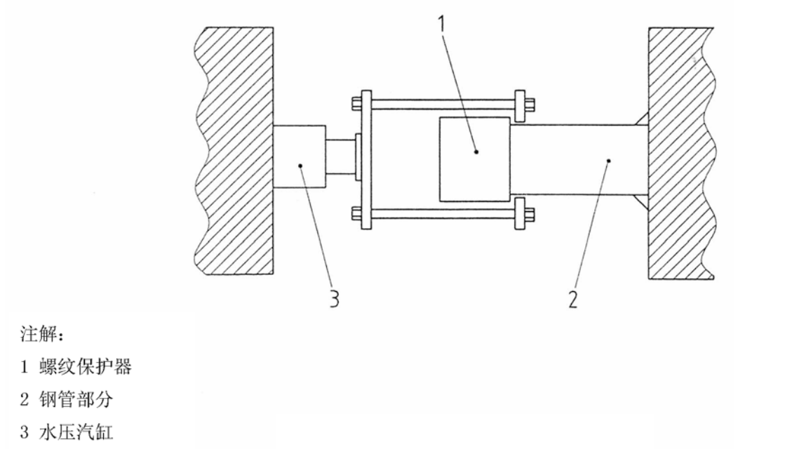
图D.29——拉脱试验装置
